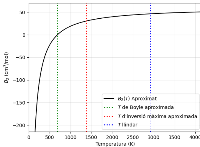
Figura 4: Representació del segon coeficient del virial aproximat a primer ordre de Taylor en funció de la temperatura, incloent-hi les posicions de la temperatura de Boyle ( T_B ) i la temperatura d'inversió màxima ( T_i ).
